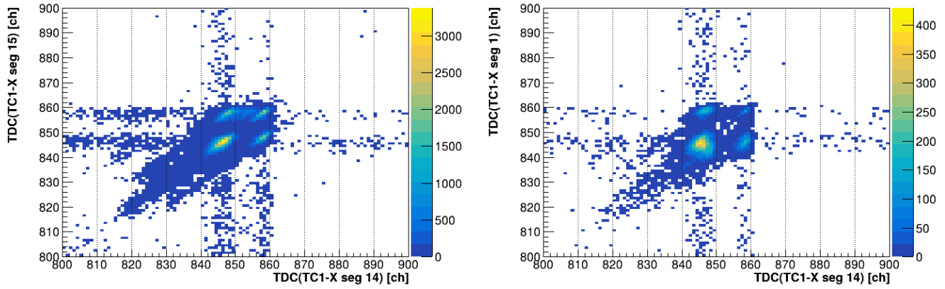
(a) TC1 X 面 セグメント 14 とセグメント 15 の TDC の二次元相関。横軸はセグメント 14 の TDC[ch]、縦軸はセグメント 15 の TDC[ch] を示す。 (b) TC1 X 面 セグメント 14 とセグメント 1 の TDC の二次元相関。横軸はセグメント 14 の TDC[ch]、縦軸はセグメント 1 の TDC[ch] を示す。
