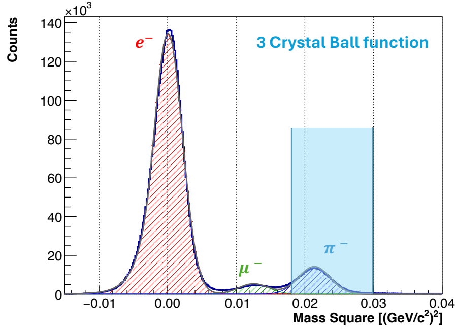
図 4.2: BH2 と TOF の間の Mass Square の分布を 3 つの Crystal Ball 関数でフィッティングした結果。横軸は Mass Square( \text{GeV}^2/c^4 )、縦軸はイベント数。水色で示した範囲がパイ中間子の選択範囲。
