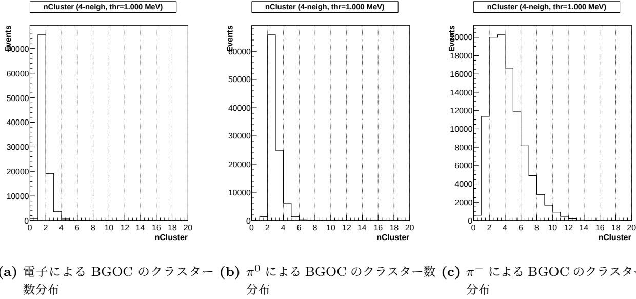
図 C.2: ビーム入射側の開口部を広げた場合の BGOC のクラスター数分布
