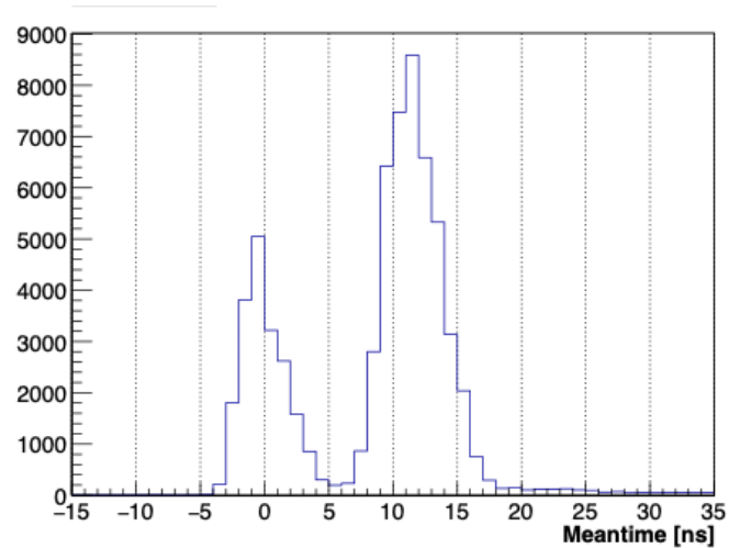
図 4.8: TC2 X 面 セグメント 13 のヒット時間分布。TDC 分布で真の hit ピークが 0 になるようオフセットされている。
