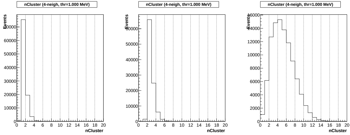
(a) Geant4 v11.2.2 で行った、電子 (b) Geant4 v11.2.2 で行った、 \pi^0 (c) Geant4 v11.2.2 で行った、 \pi^- による BGOC のクラスター数分布 による BGOC のクラスター数分布 による BGOC のクラスター数分布
