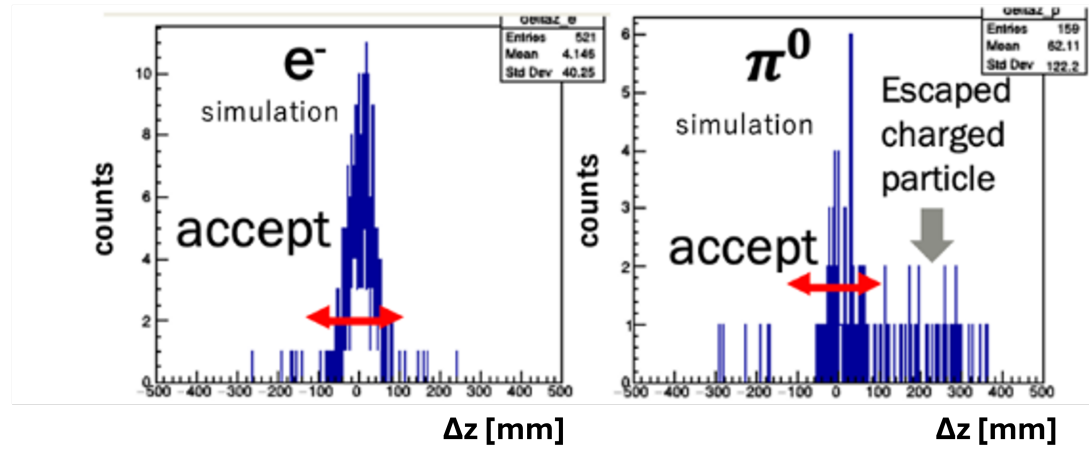
図 2.5: BGOC と TH のヒット位置の z 座標差 \Delta z の分布例。
