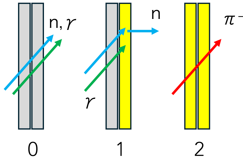
図4.12: Veto Counterのmultiplicityの概念図。各ペアの両方がヒットした場合、multiplicityは2となり、そのイベントは除去される。
