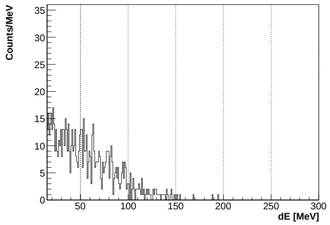
(d) 実験データでの BGO2 のエネルギースペクトル。15 MeV を始点とする。
