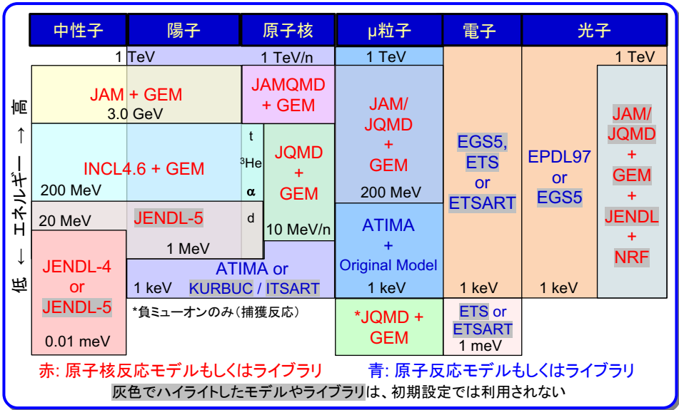
図 5.14: PHITS で使用される主要な物理モデルの概要 [72]。
