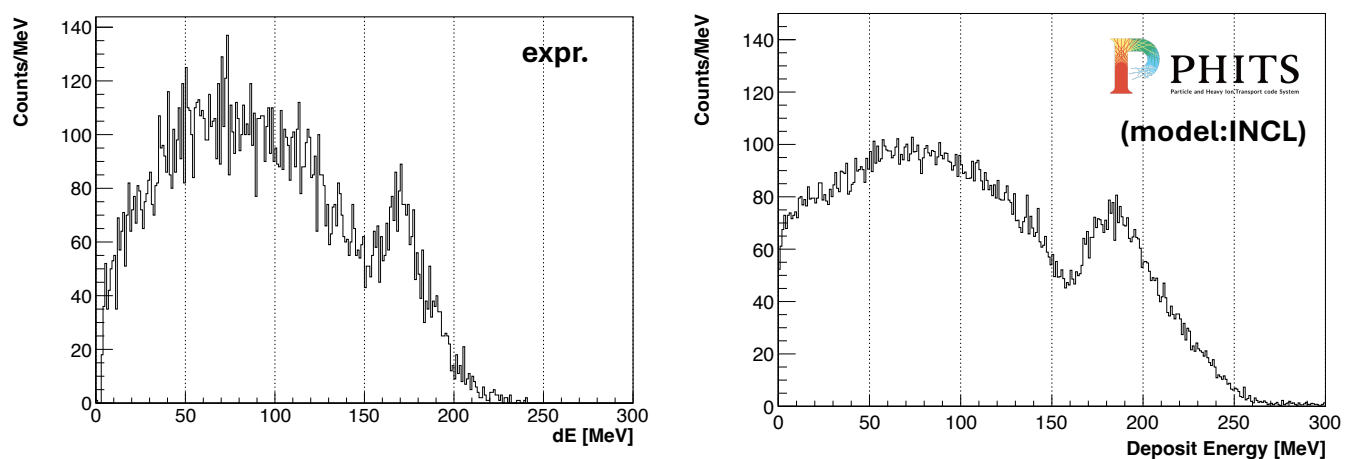
図 5.21: BGO1 のエネルギースペクトルの実験データ (左) と PHITS シミュレーション結果 (右) の比較。横軸がエネルギー (MeV)、縦軸が事象数。
