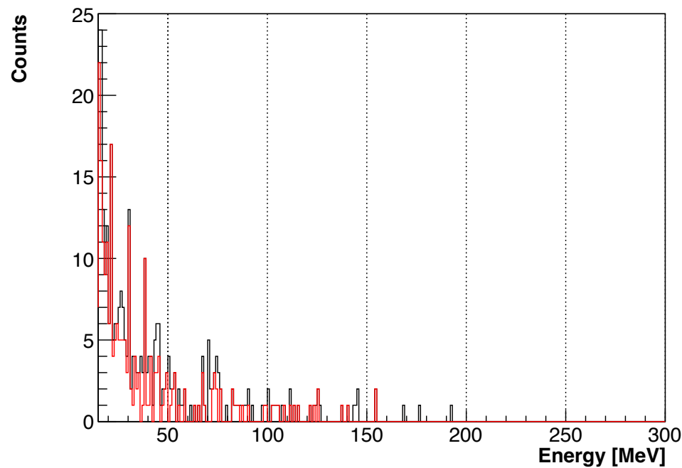
図 5.9: INCL モデルを用いた Geant4 シミュレーションによる BGO2 のエネルギースペクトル。横軸がエネルギー (MeV)、縦軸が事象数。横軸の範囲は 15 MeV から 300 MeV まで。黒が粒子種を問わない全成分、赤が中性子によるヒット成分。
