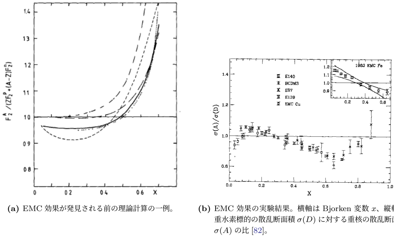
図 B.1: EMC 効果の理論計算と実験結果の比較。
