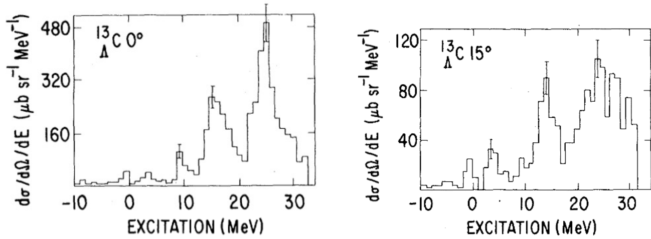
(a) ^{13}\text{C}(K^-, \pi^-)^{13}_{\Lambda}\text{C} の生成断面積 (散乱角 \theta = 0^\circ の場合) [26]。 (b) ^{13}\text{C}(K^-, \pi^-)^{13}_{\Lambda}\text{C} の生成断面積 (散乱角 \theta = 15^\circ の場合) [26]。
