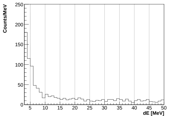
(f) 実験データでの BGO2 のエネルギースペクトル。3 MeV を始点とする。
