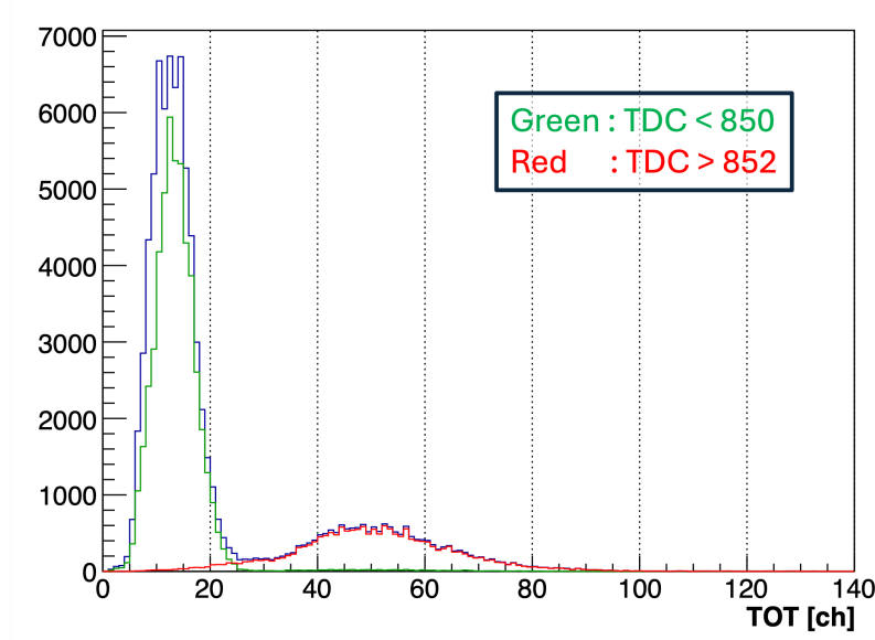
図 4.6: TC2 X 面 セグメント 13 の TOT 分布。横軸は TOT[ch]、縦軸はイベント数を示す。
