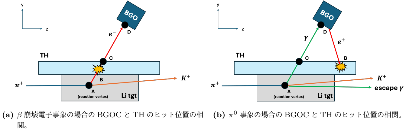
図 2.4: BGOC と TH のヒット位置の相関の例。
