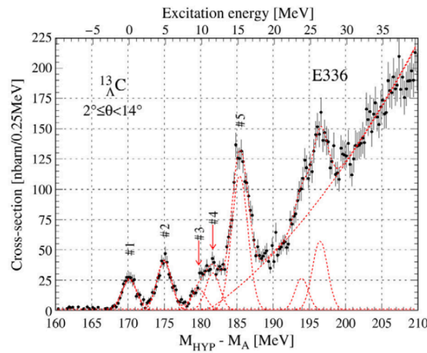
(c) ^{13}\text{C}(\pi^+, K^+)^{13}_{\Lambda}\text{C} の生成断面積, [24] による図を引用。データの詳細は [25] を参照。
