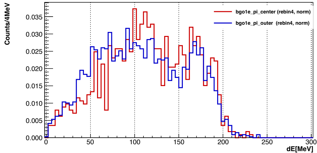
図 4.30: BGO1 エネルギースペクトルの位置依存性比較。赤ヒストグラムは中心領域（ |x| < 10 mm かつ |y| < 10 mm）、青ヒストグラムは外側領域（ |x| < 20 mm, |y| < 20 mm, \max(|x|, |y|) \geq 10 mm）を表す。それぞれのヒストグラムのエントリー数を 1 とした規格化分布（縦軸: Counts/4 MeV）である。横軸は BGO1 dE [MeV]。
