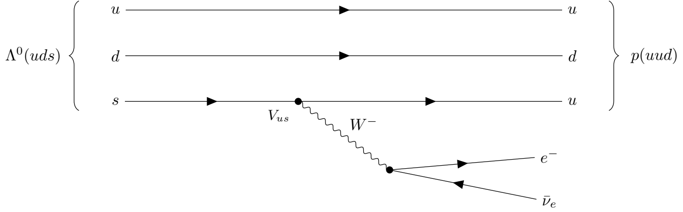
図 A.1: \Lambda \rightarrow p e^- \bar{\nu}_e 崩壊のファインマン図 (クォークレベル)。ストレンジクォークが弱相互作用によりアップクォークへ遷移する。他の u, d クォークはスペクテーターとして振る舞う。
